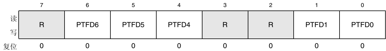
图 6-33. F 口数据寄存器（PTFD）
