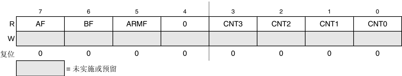
图 15-9. 调试状态寄存器 (DBGS)
