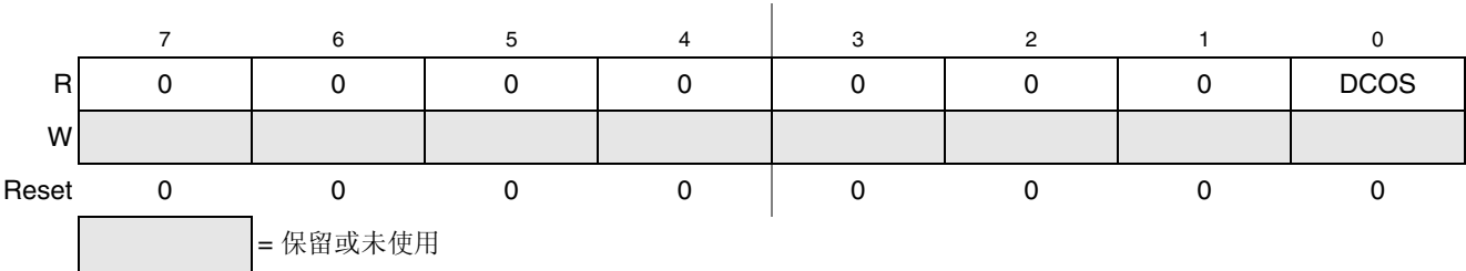
图 9-9. ICG 状态寄存器 2（ICGS2）
