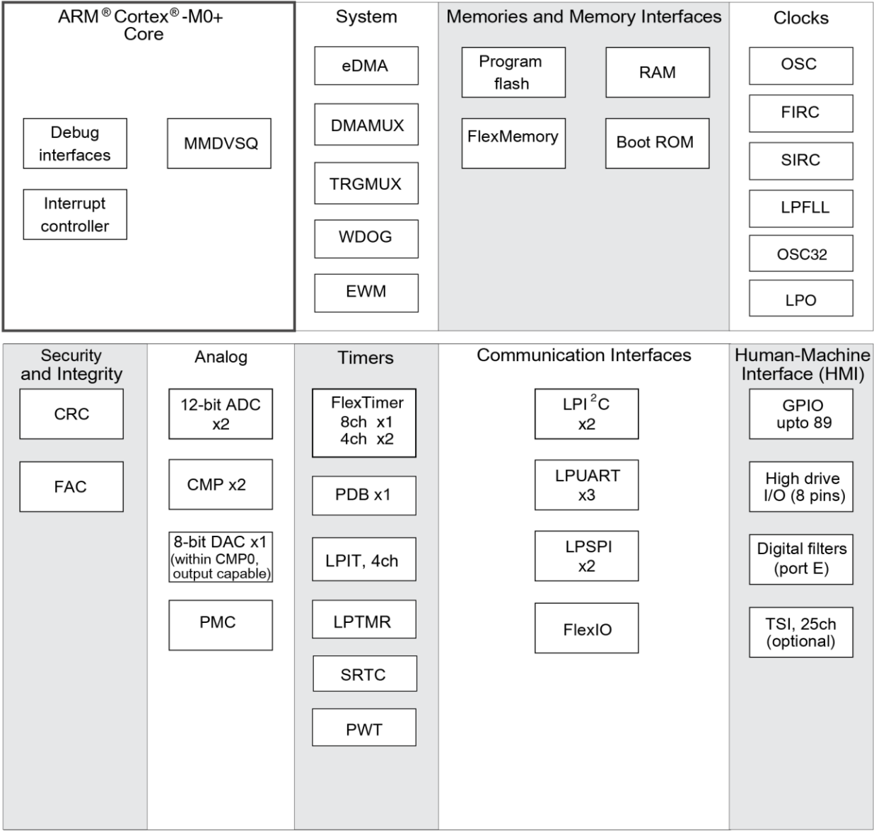
图 1.功能框图
