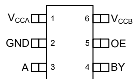
图 4-2. DCK 封装，6 引脚 SC70 透明 (顶视图)
