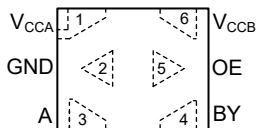
图 4-5. DTQ 封装，6 引脚 X2SON 透明 (顶视图)
