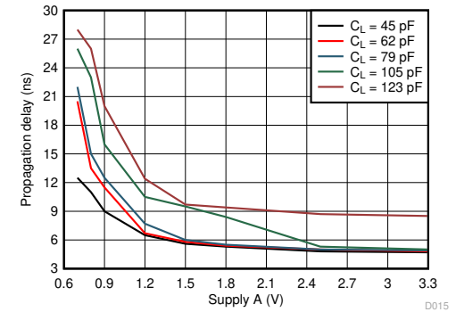
图 5-14. 从低电平转换到高电平的典型传播延迟 (B 到 A) 与负载电容间的关系
