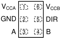
图 4-2. DRY 封装，6 引脚 SON 透明（顶视图）
