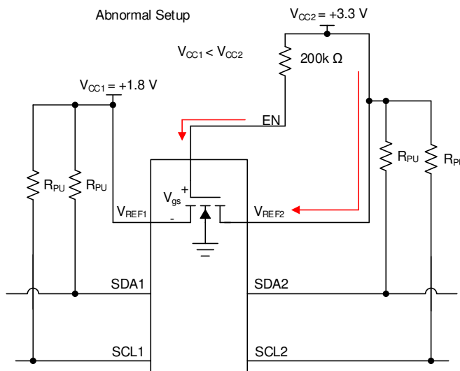
图 8-2. Abnormal Setup
