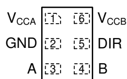
图 5-4. DRY Package 6-Pin SON Transparent Top View
