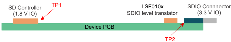
图 11-2. 器件放置
