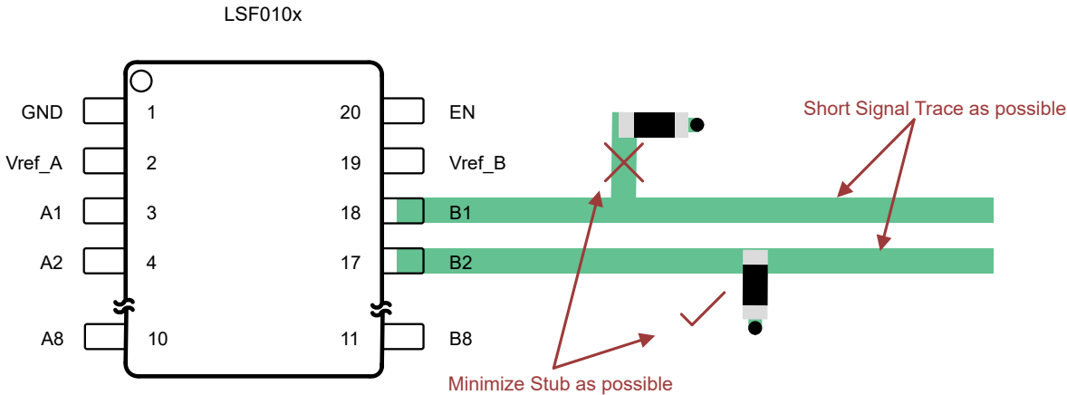
图 11-1. 短布线布局
