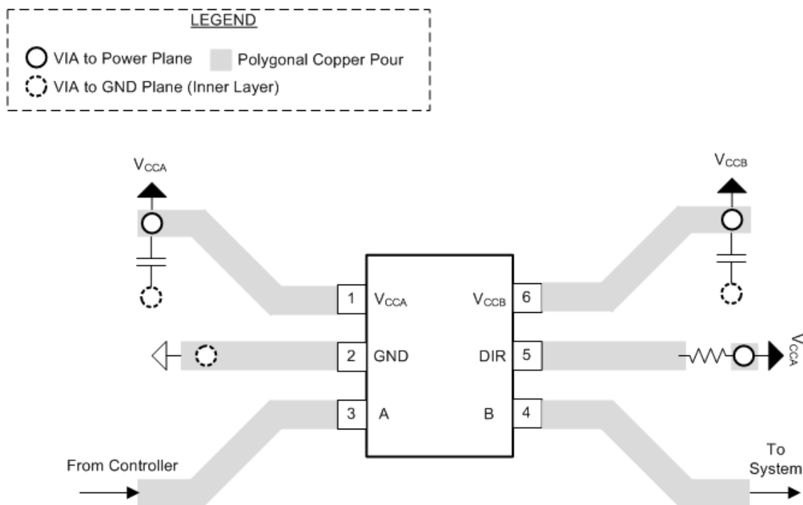
图 9-1. Layout Schematic
