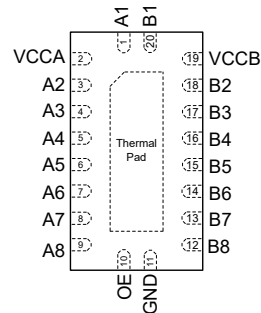
图 4-2. RKS 封装，20 引脚 VQFN（顶视图）
