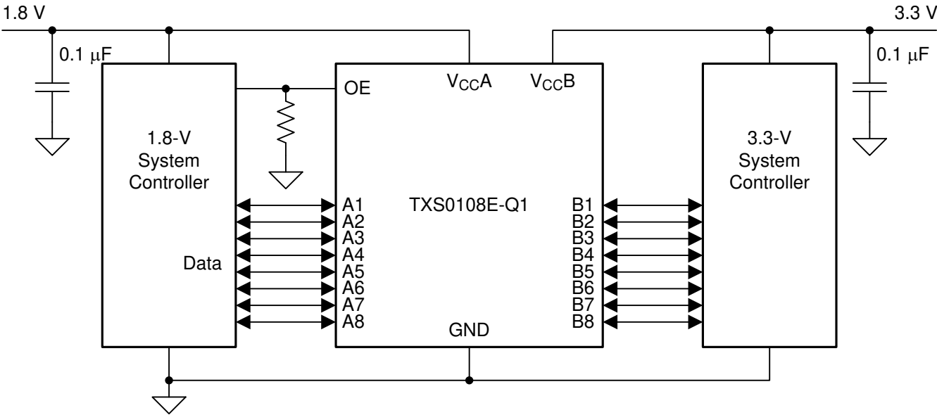
图 8-1. 典型应用电路
