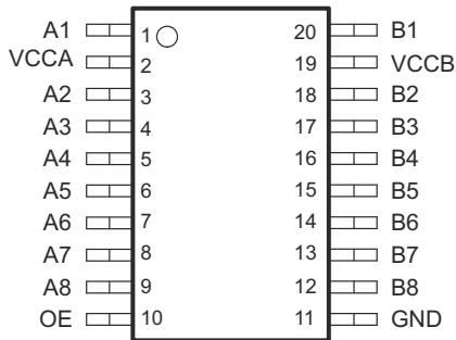
图 4-1. PW 封装，20 引脚 TSSOP（顶视图）
