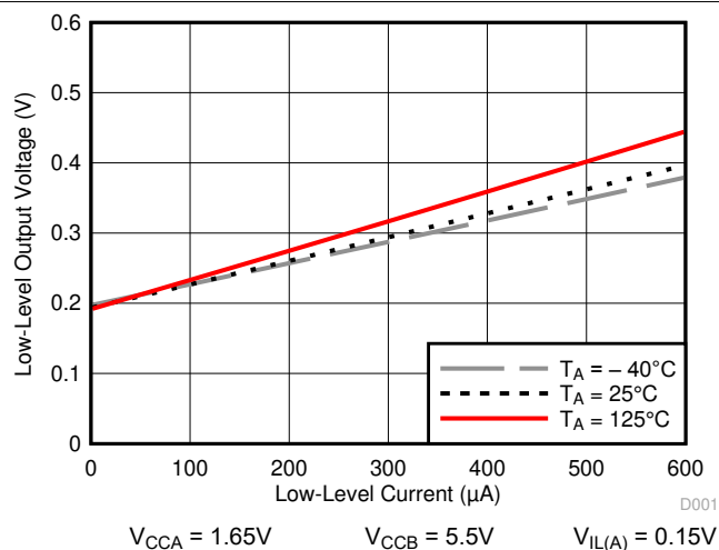
图 5-4. 低电平输出电压 ( V_{OL(Bx)} ) 与低电平电流 ( I_{OL(Bx)} ) 间的关系
