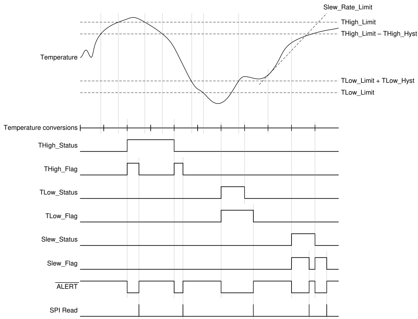
图 8-7. 中断模式图
