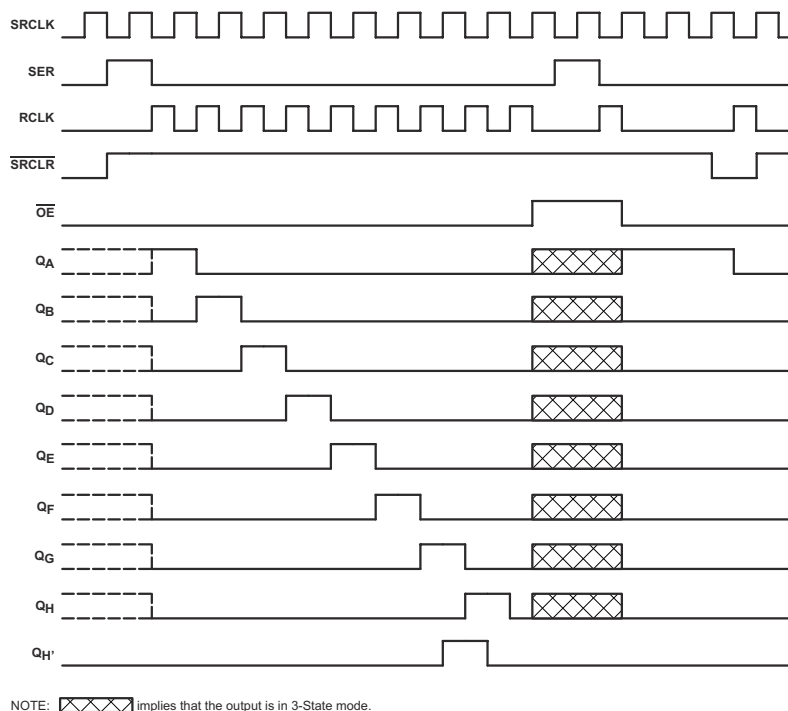
图 5-1. 时序图
