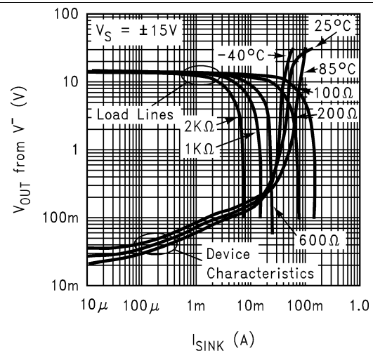
图 60. 输出灌电流特性以及负载线
