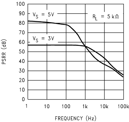
图 5-17. 负 PSRR 与频率间的关系
