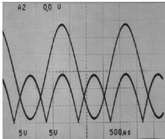
图 7-20. 全波整流器波形
