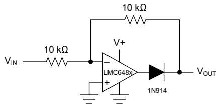
图 7-17. 具有输入电流保护 ( R_i ) 的半波整流器
