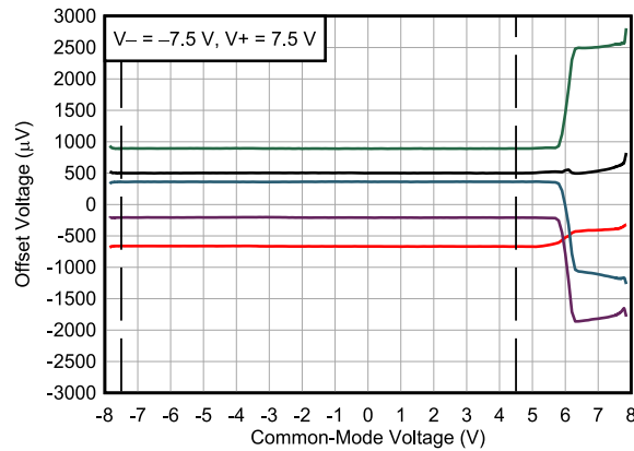
图 6-1. 输入失调电压与共模电压间的关系
