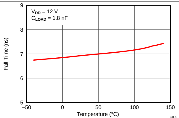
图 12. Fall Time vs Temperature
