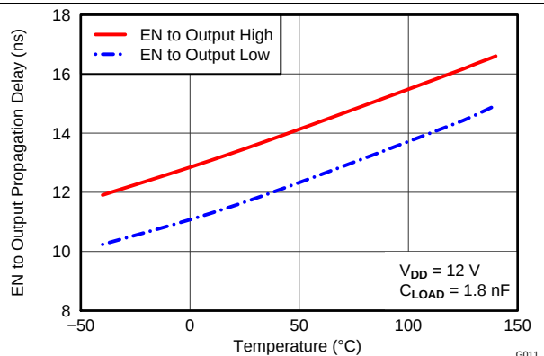
图 14. En to Output Propagation Delay vs Temperature
