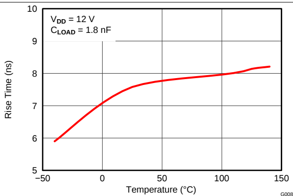
图 11. Rise Time vs Temperature
