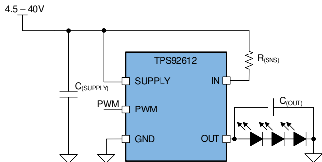
典型应用图
