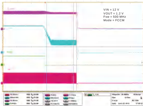
图 31. Overcurrent Protection
