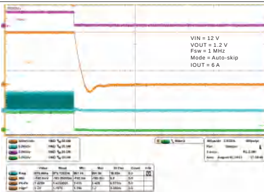
图 27. Shutdown Operation
