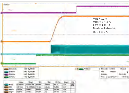
图 23. Start-Up
