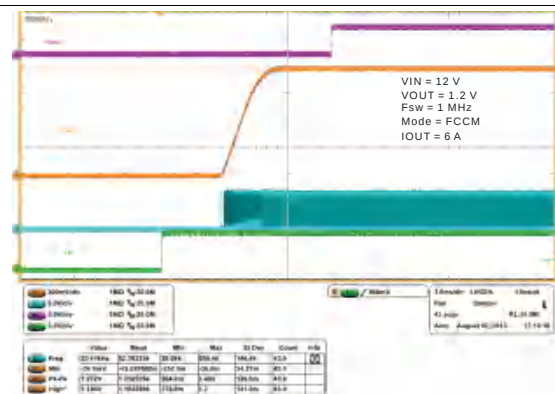
图 24. Start-Up
