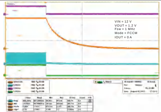
图 26. Shutdown Operation
