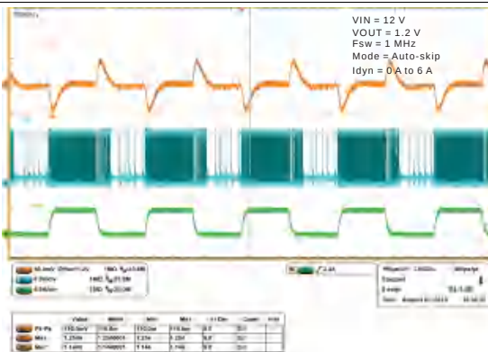
图 19. Auto-Skip Mode Load Transient
