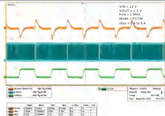
图 20. FCCM Mode Load Transient
