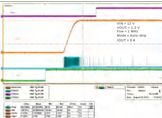
图 21. Start-Up
