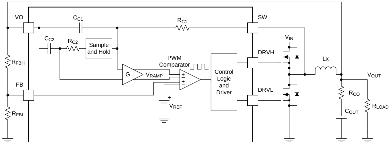
图 40. D-CAP3 Mode
