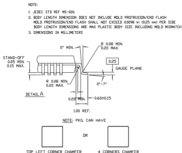
图 21. 100 引脚 TQFP (14 × 14 × 1.4 mm) A100SA 封装外形, 51-85048
