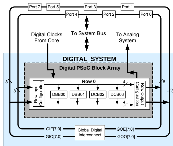
图 2. 数字系统框图
