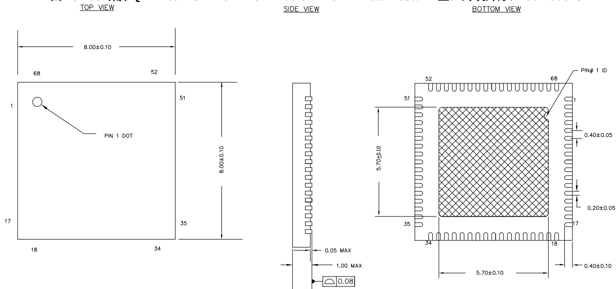
图 19. 68 引脚 QFN ( 8 \times 8 \times 1.0 mm) LT68 5.7 \times 5.7 E-Pad (Sawn 型) 封装外形, 001-09618
