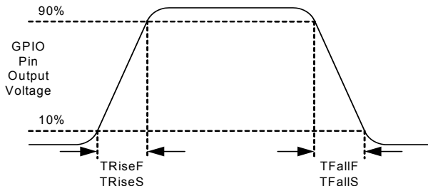
图 12. GPIO 时序图
