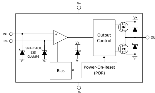
TLV903x-Q1 方框图
