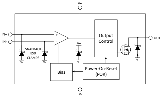
TLV902x-Q1 方框图
