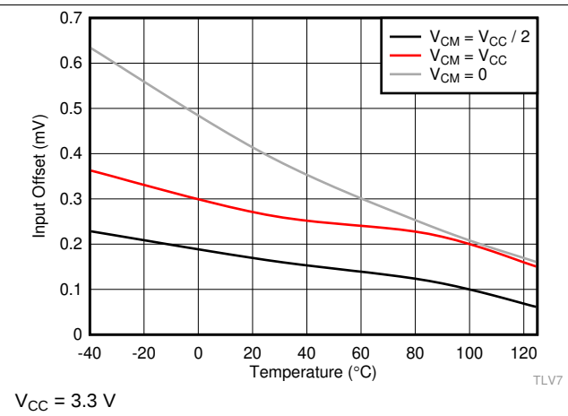
图 16. Input Offset vs. Temperature
