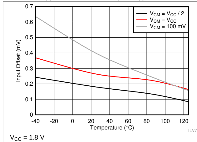
图 15. Input Offset vs. Temperature
