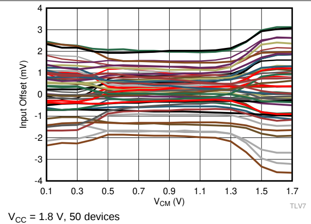
图 18. Input Offset Voltage vs. V_{CM}
