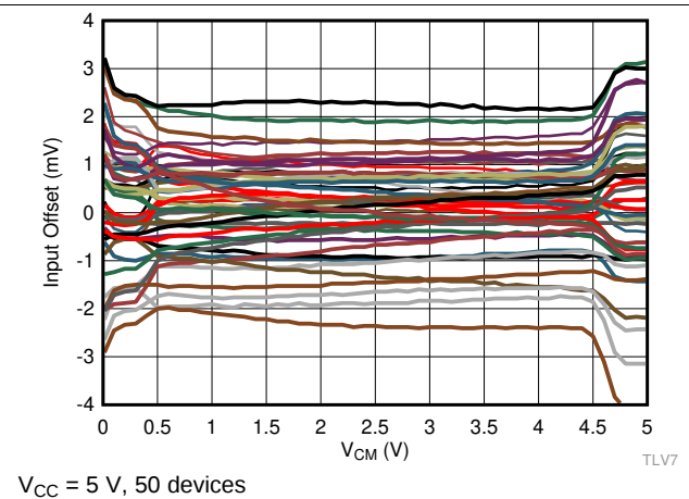
图 20. Input Offset Voltage vs. V_{CM}
