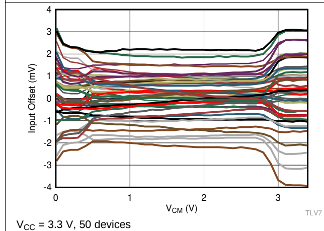
图 19. Input Offset Voltage vs. V_{CM}
