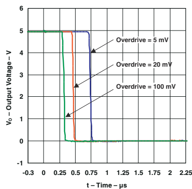
图 6-4. 负转换时各种过驱的响应时间
