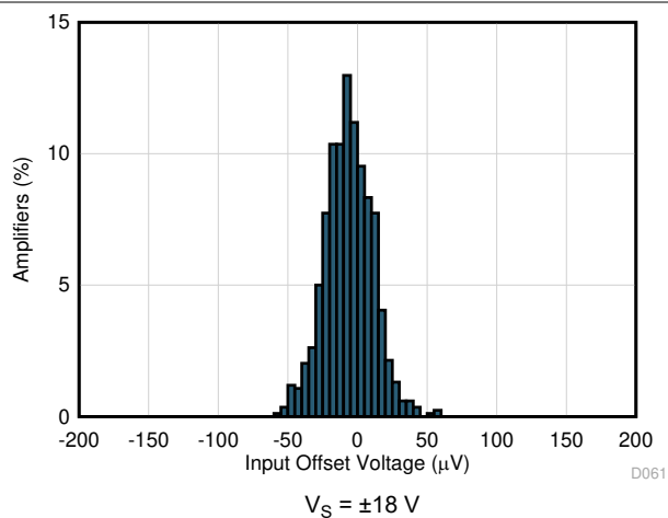
图 6-14. Input Offset Voltage Histogram
