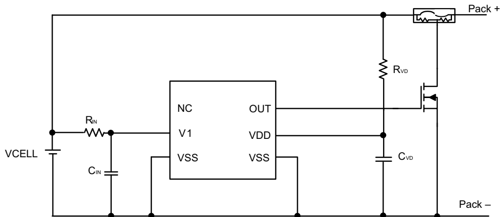
简化原理图
