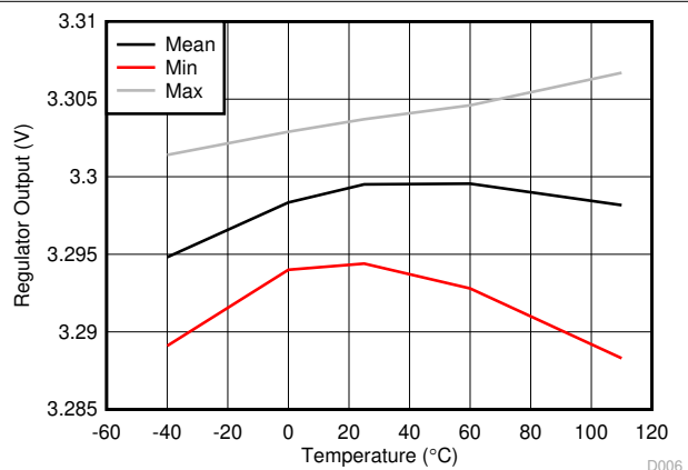
图 7-6. Regulator Output Without Load
