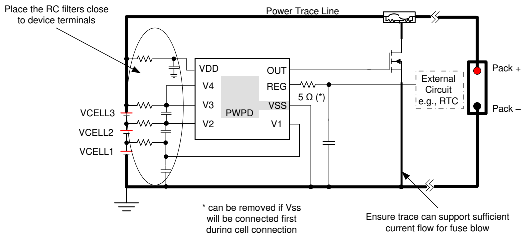
图 11-1. Layout Example
