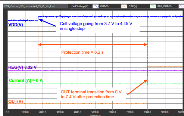
图 9-4. Overvoltage Protection
