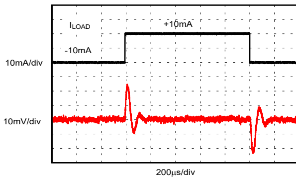
图 7-20. 负载瞬态
