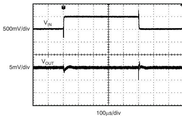
图 7-22. 线路瞬态
