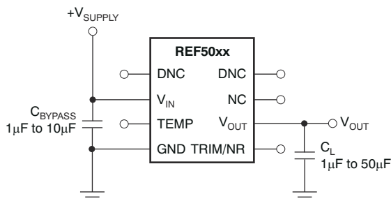
图 9-4. 基本连接
