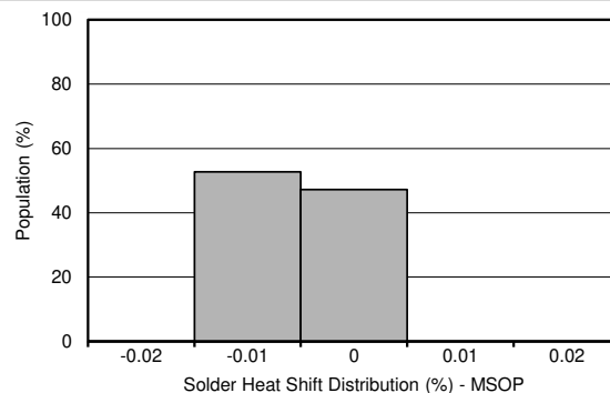
图 8-3. 焊接热移位分配 (%), VSSOP 封装
