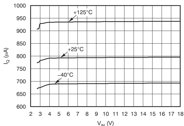
图 7-10. 静态电流与输入电压间的关系
