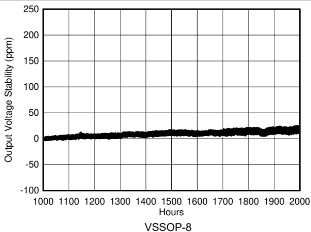
图 7-24. REF50xx 长期稳定性 (后 1000 小时)
