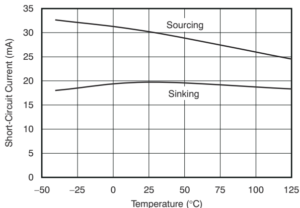
图 7-12. 短路电流与温度间的关系
