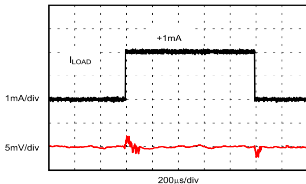
图 7-19. 负载瞬态
