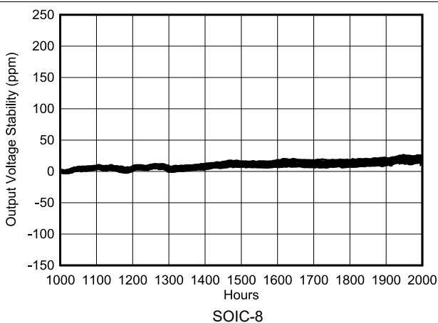
图 7-29. REF50xx 长期稳定性 (后 1000 小时)
