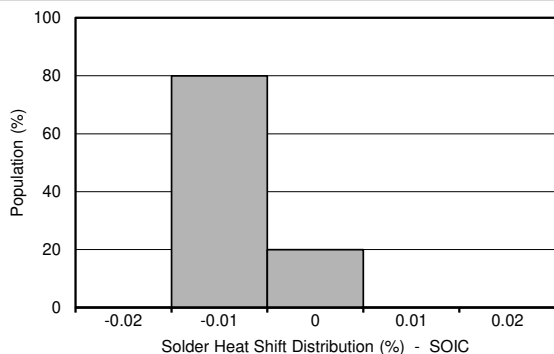
图 8-2. 焊接热移位分配 (%), SOIC 封装
