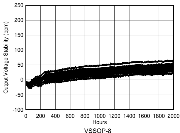
图 7-25. REF50xx 长期稳定性 (前 2000 小时)
