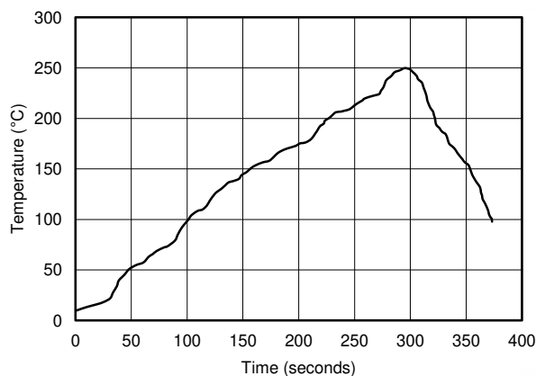
图 8-1. 回流焊曲线
