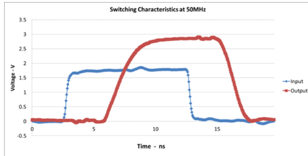
图 7-1. 出色的信号完整性 ( 3.3V V_{CC} 时为 1.8V 至 3.3V )
