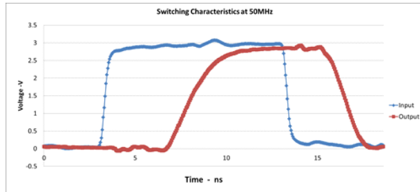
图 7-2. 出色的信号完整性 ( 3.3V V_{CC} 时为 3.3V 至 3.3V )
