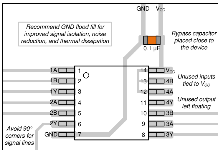
图 10-1. SN74LV1T32 的示例布局
