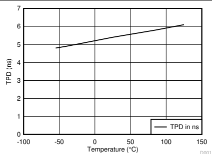
图 6-1. TPD vs Temperature
