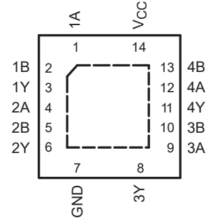
图 5-2. SN74AHC132 RGY Package, 14-Pin VQFN (Top View)
