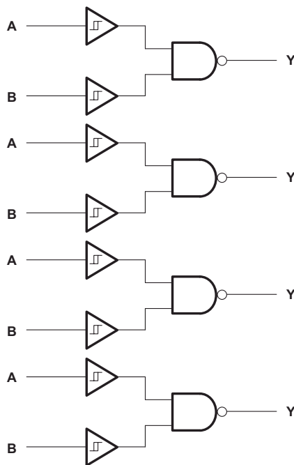
简化版电路原理图
