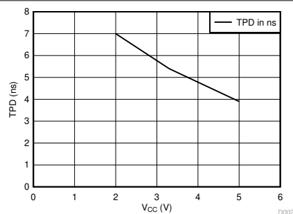
图 6-2. TPD vs VCC
