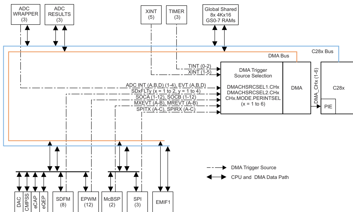
图 8-3. DMA 方框图
