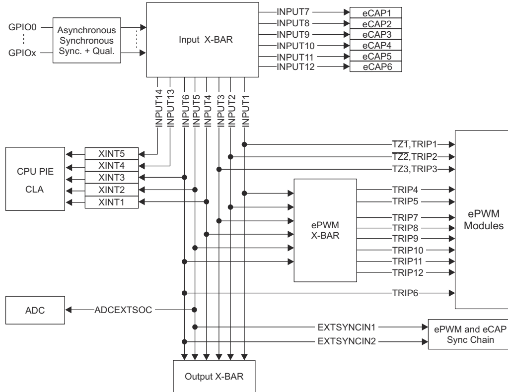
图 6-3. 输入 X-BAR
