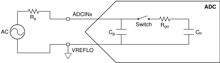
图 7-31. 单端输入模型
