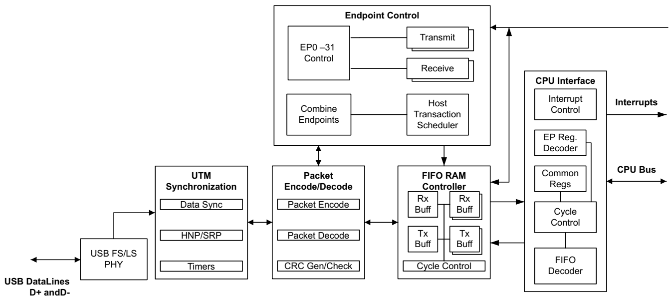
图 7-72. USB 方框图
