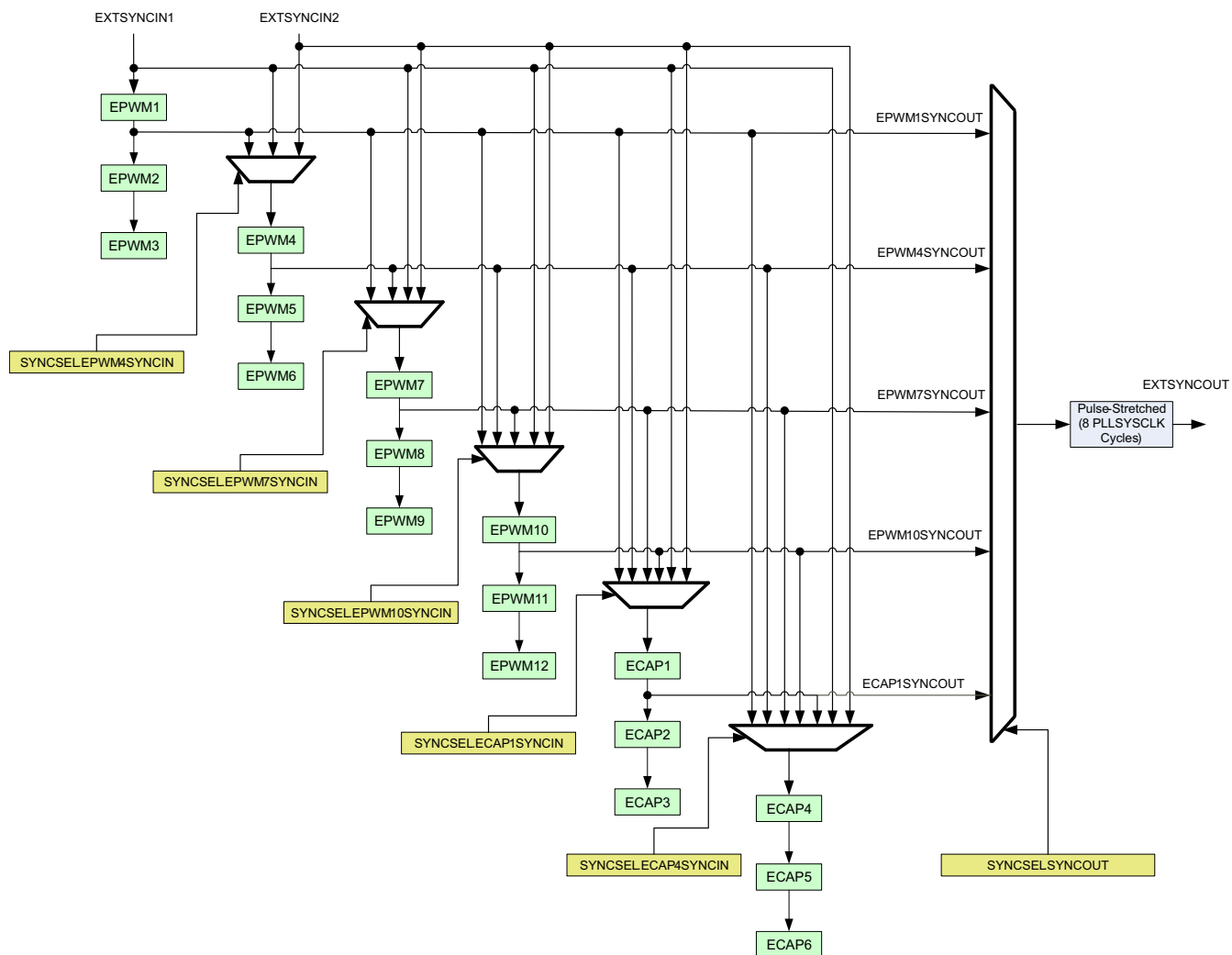
图 7-47. 同步链架构
