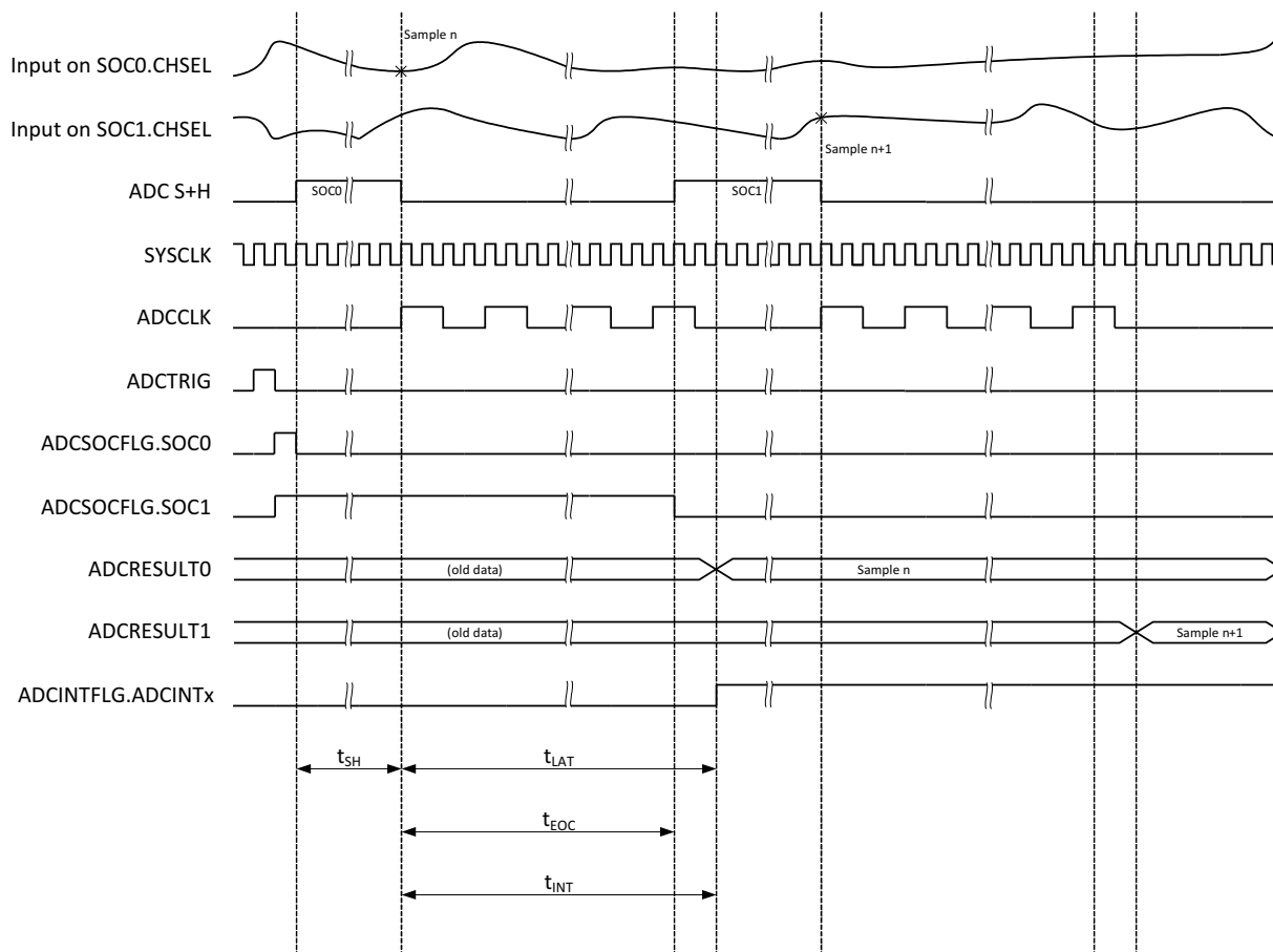
图 7-32. 12 位模式的 ADC 时序
