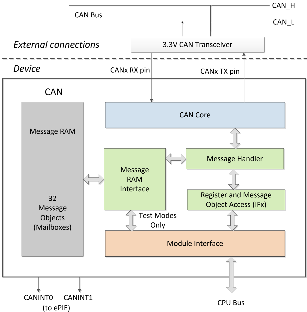
图 7-56. CAN 方框图
