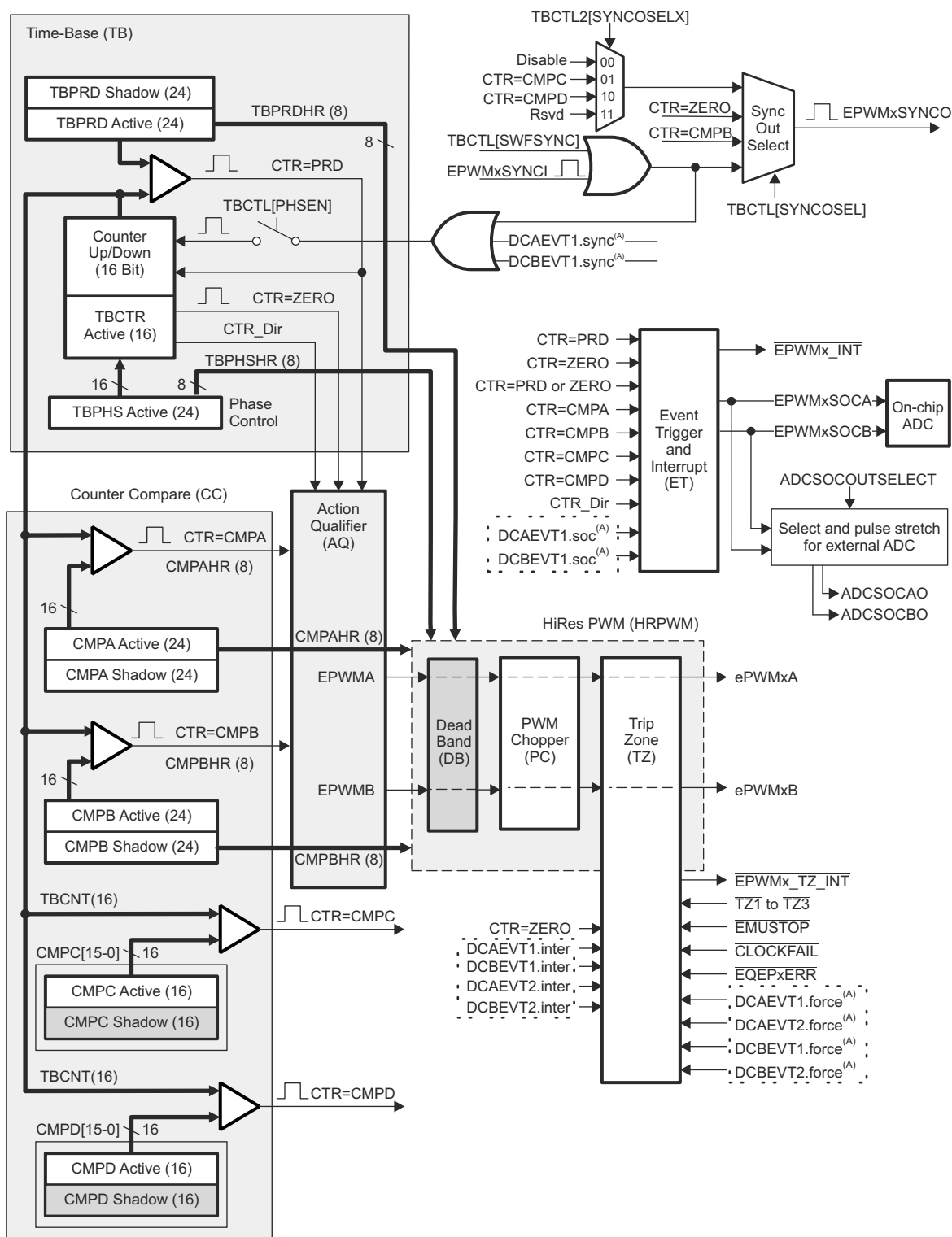
图 7-45. ePWM 子模块和关键内部信号互连
