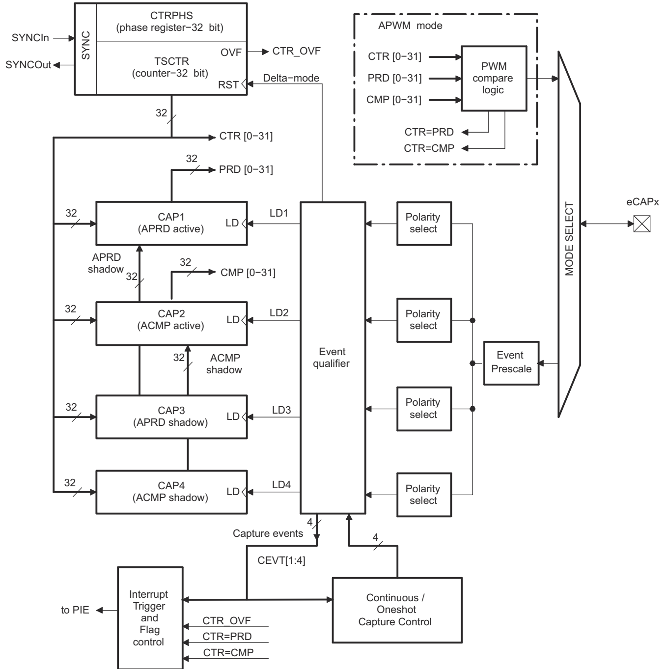
图 7-44. eCAP 方框图
