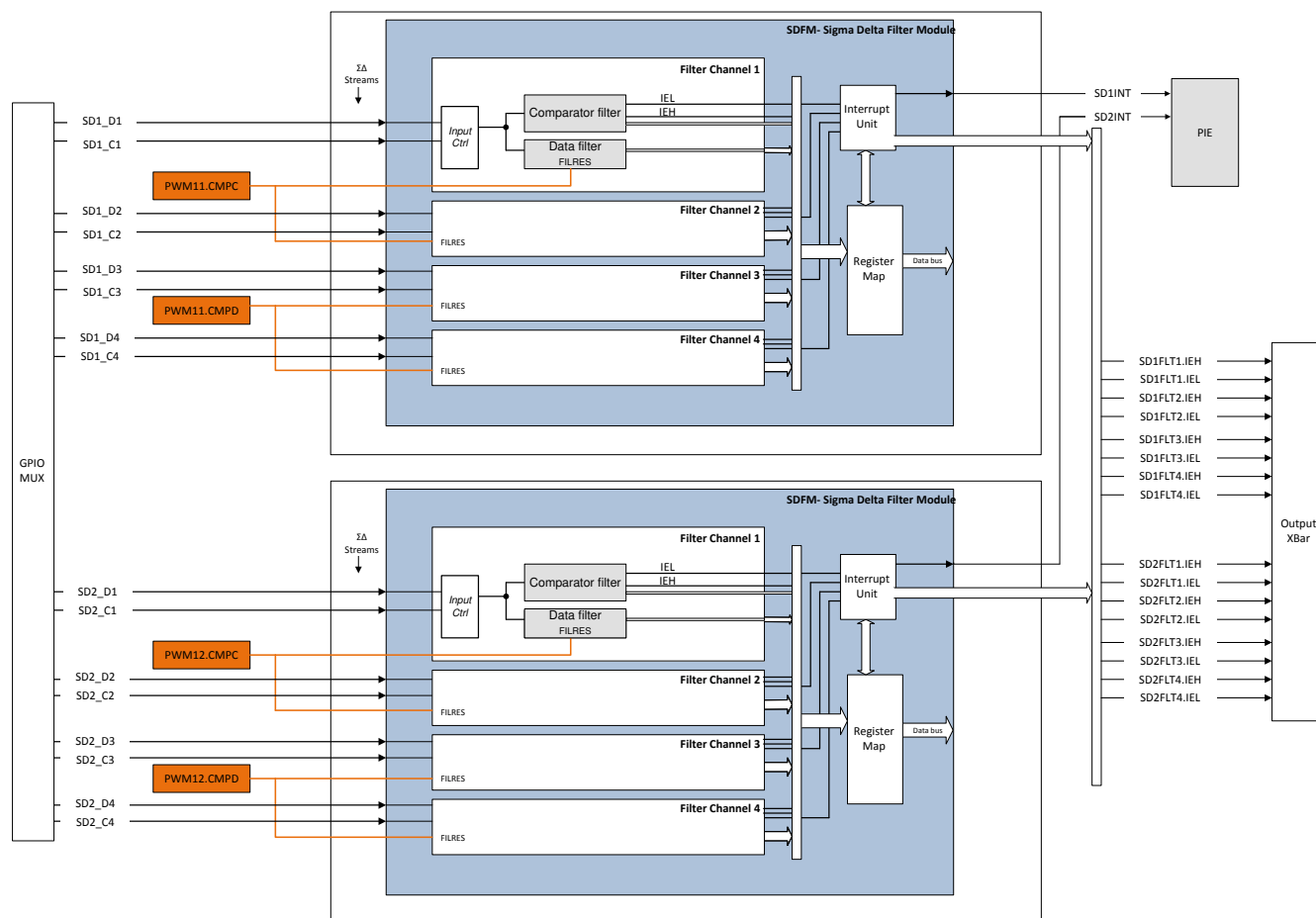
图 7-51. SDFM 方框图
