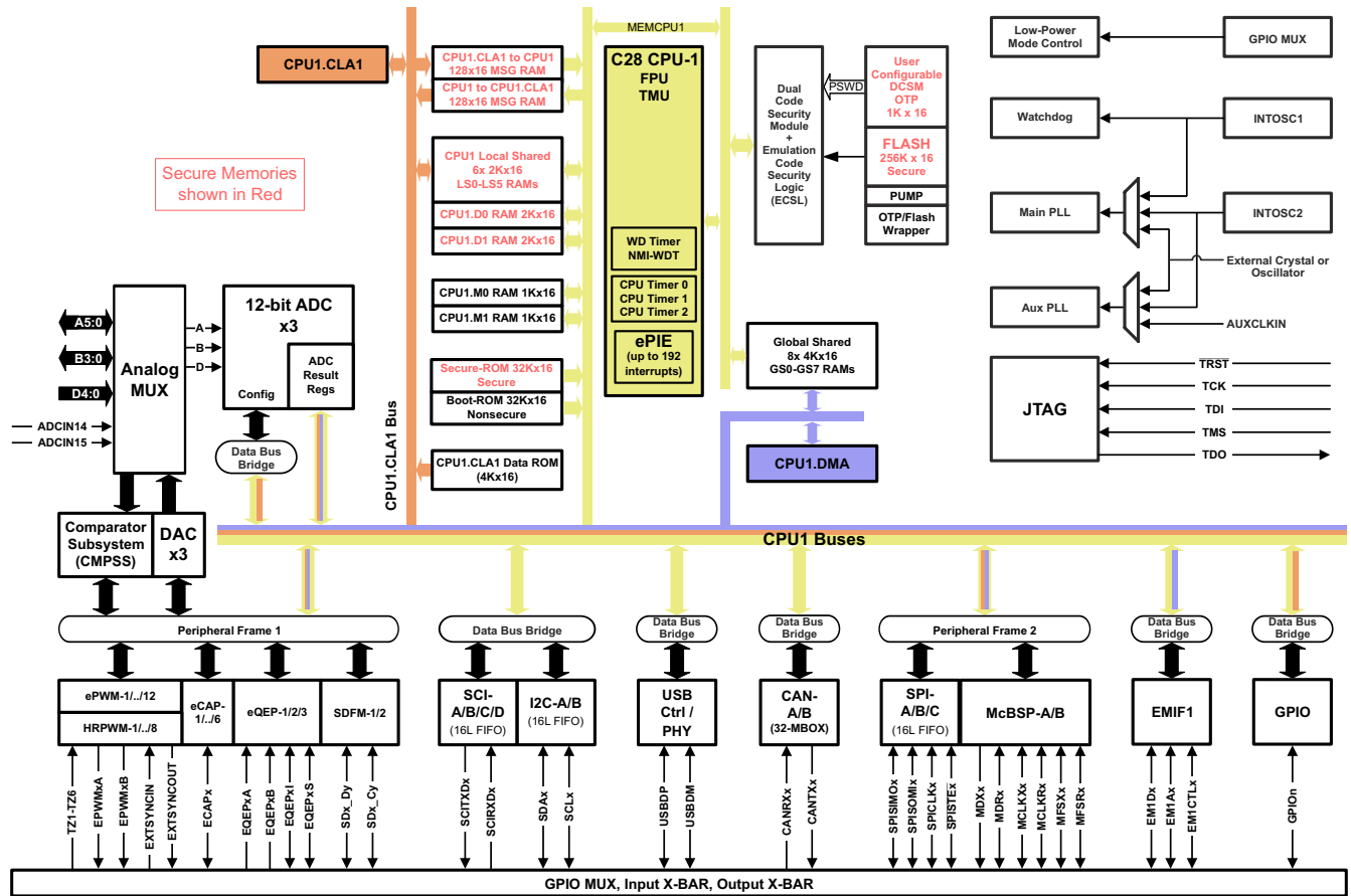
图 8-1. 功能方框图
