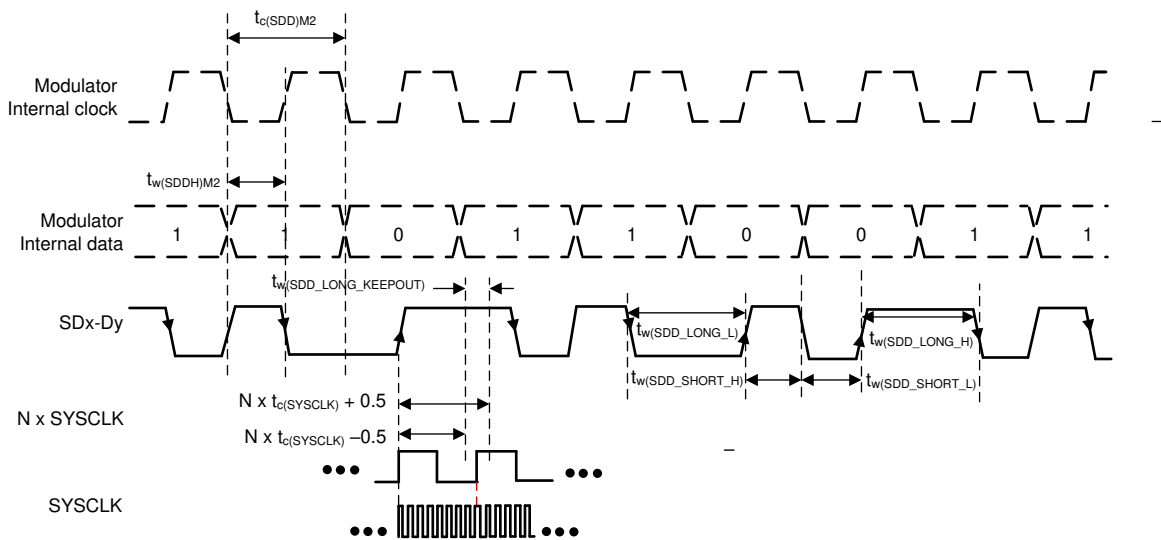
图 7-54. SDFM 时序图 - 模式 2
