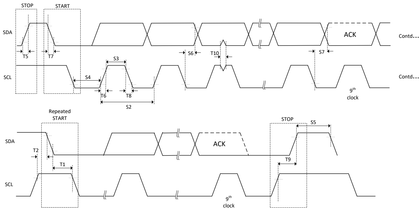
图 7-58. I2C 时序图
