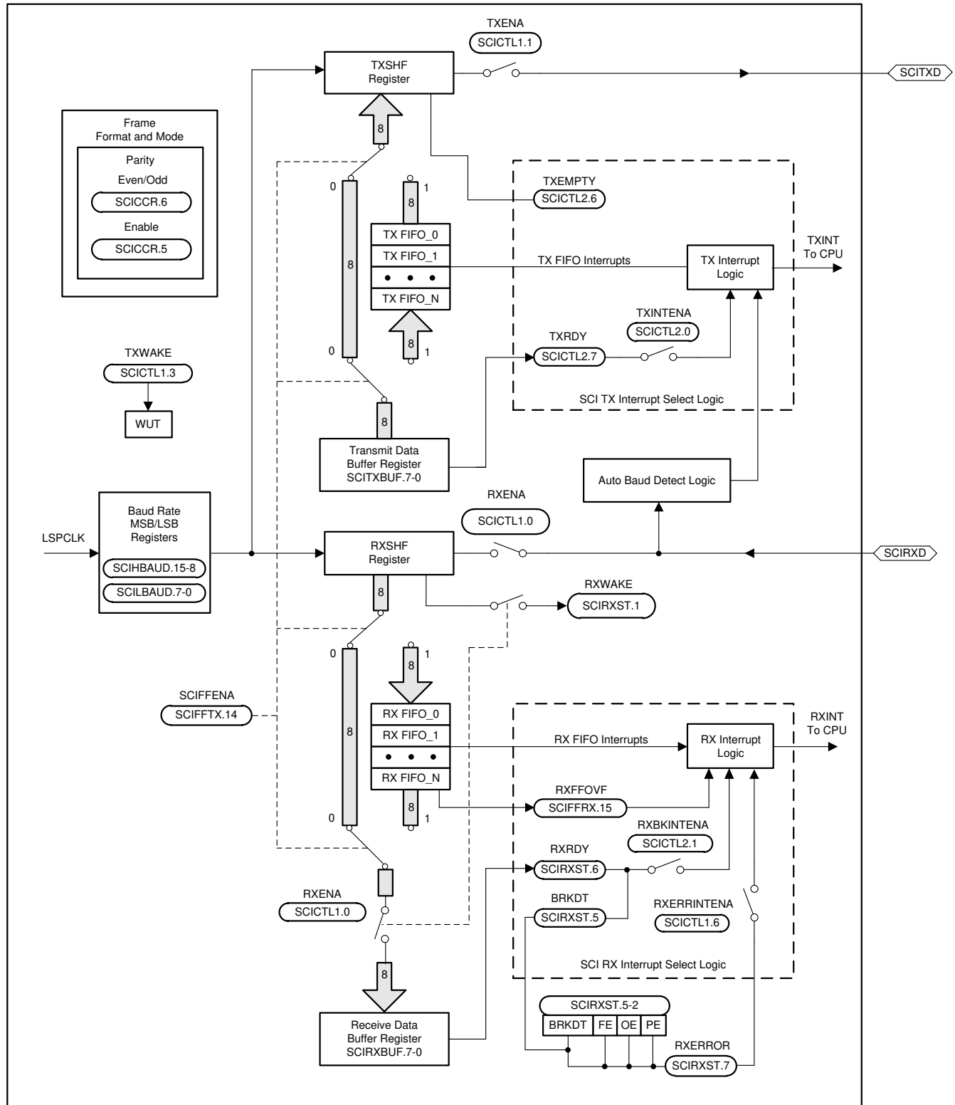
图 7-66. SCI 方框图
