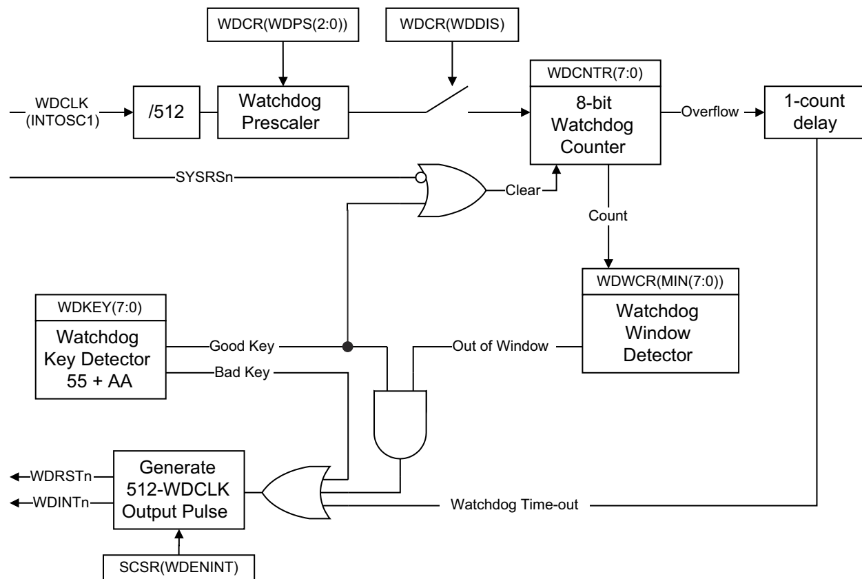
图 8-4. 窗口看门狗
