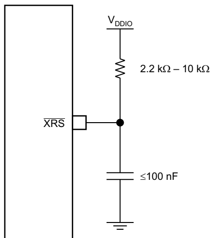
图 7-4. 复位电路
