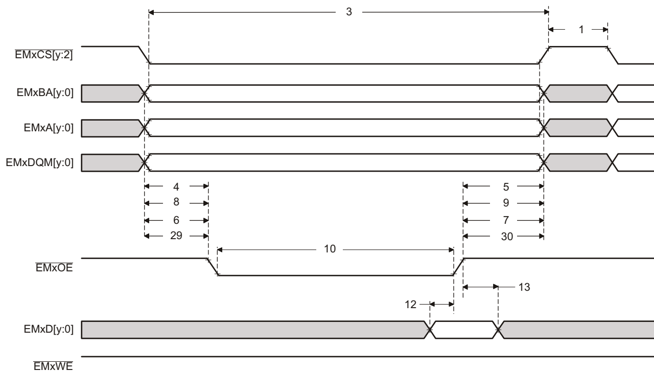
图 7-21. 异步存储器读取时序
