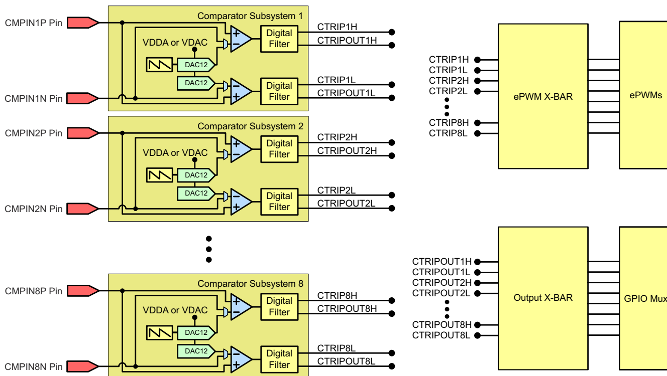
图 7-33. CMPSS 连接 ( 176 引脚 PTP )
