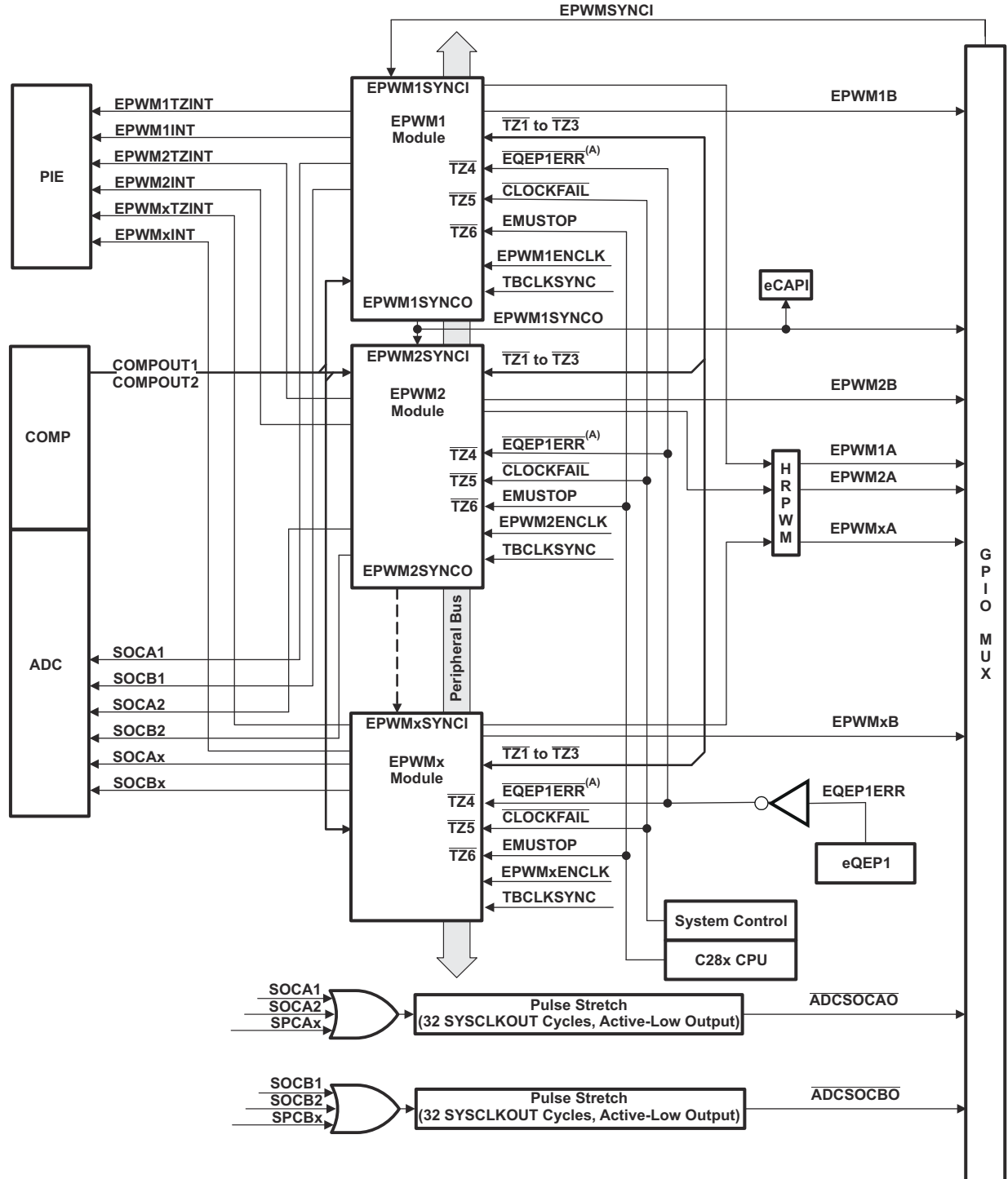
图 8-48. ePWM
