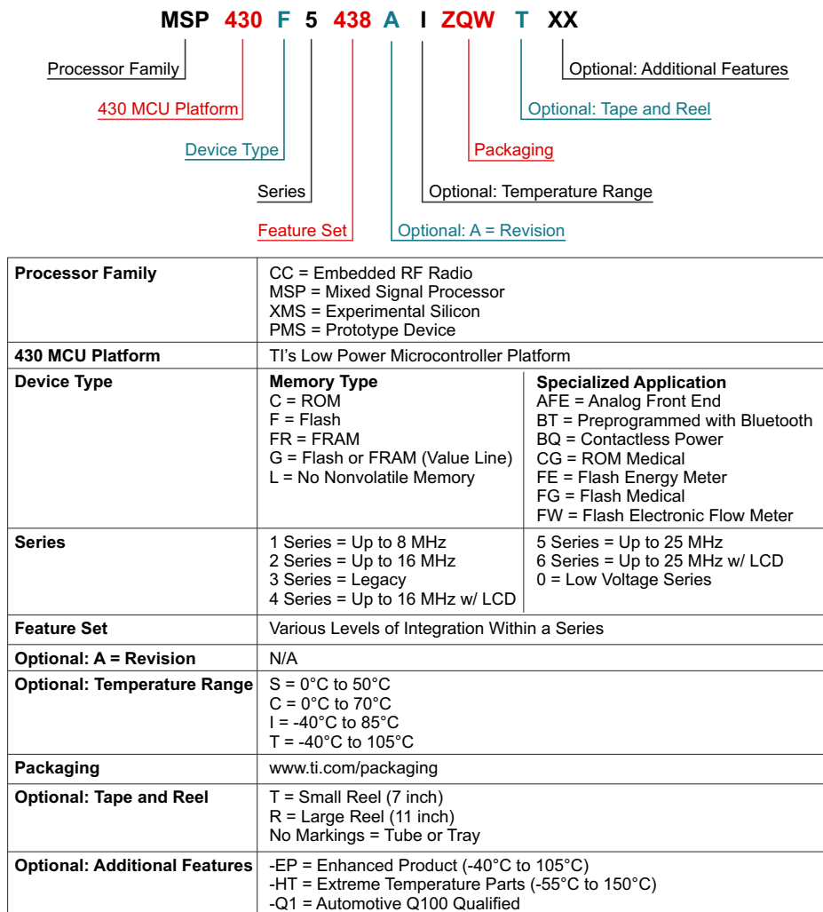
图 7-1. 器件命名规则
