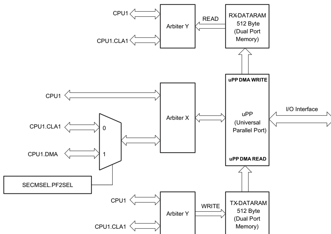
图 8-77. uPP 集成
