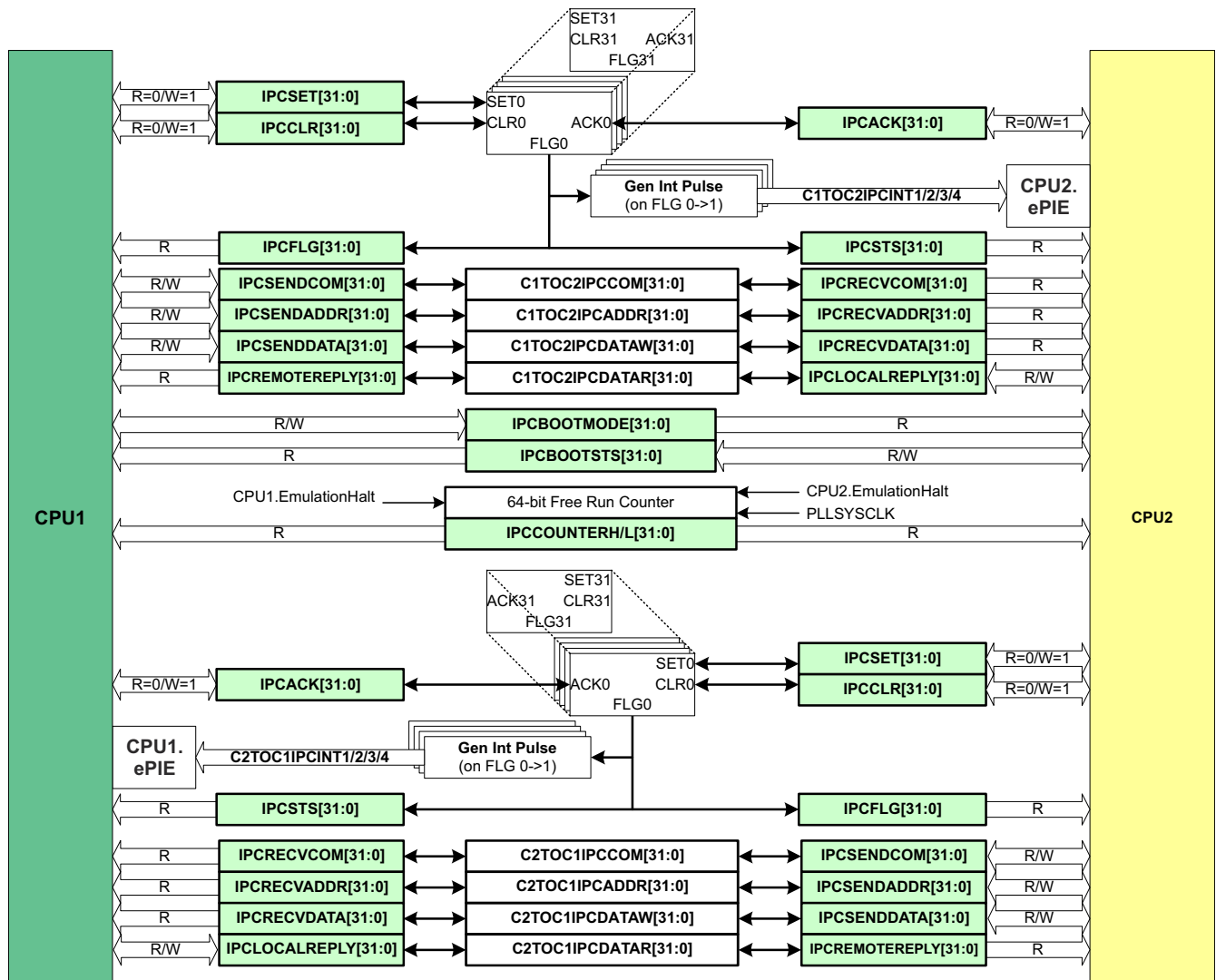
图 9-4. IPC 架构
