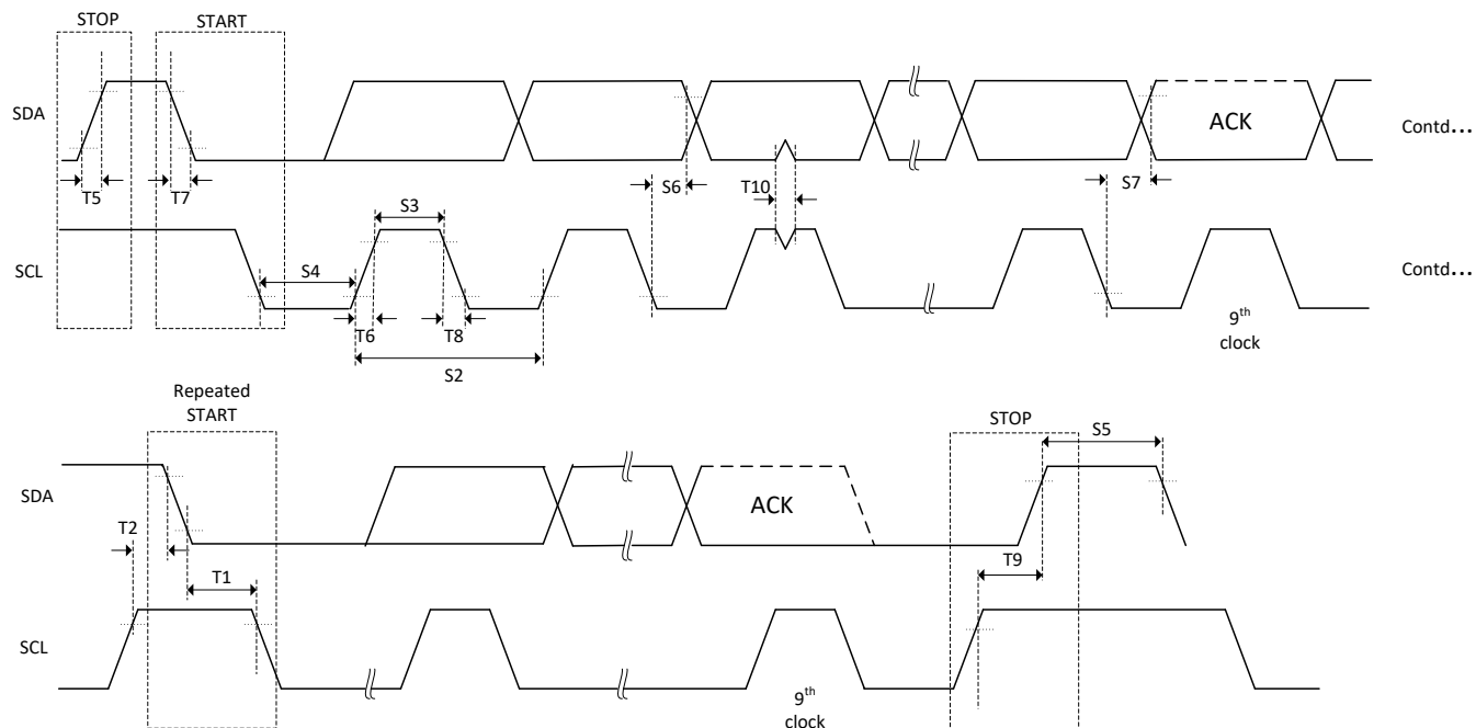
图 8-62. I2C 时序图
