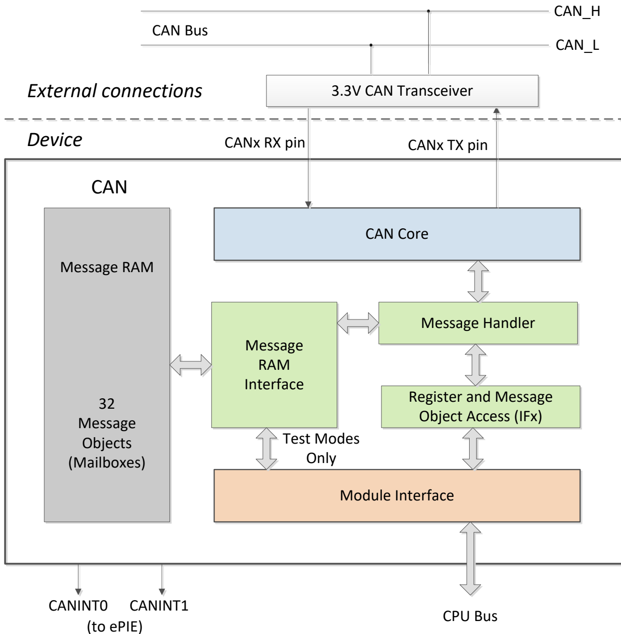
图 8-60. CAN 方框图
