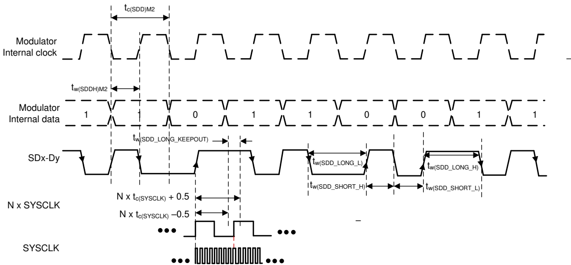
图 8-58. SDFM 时序图 - 模式 2
