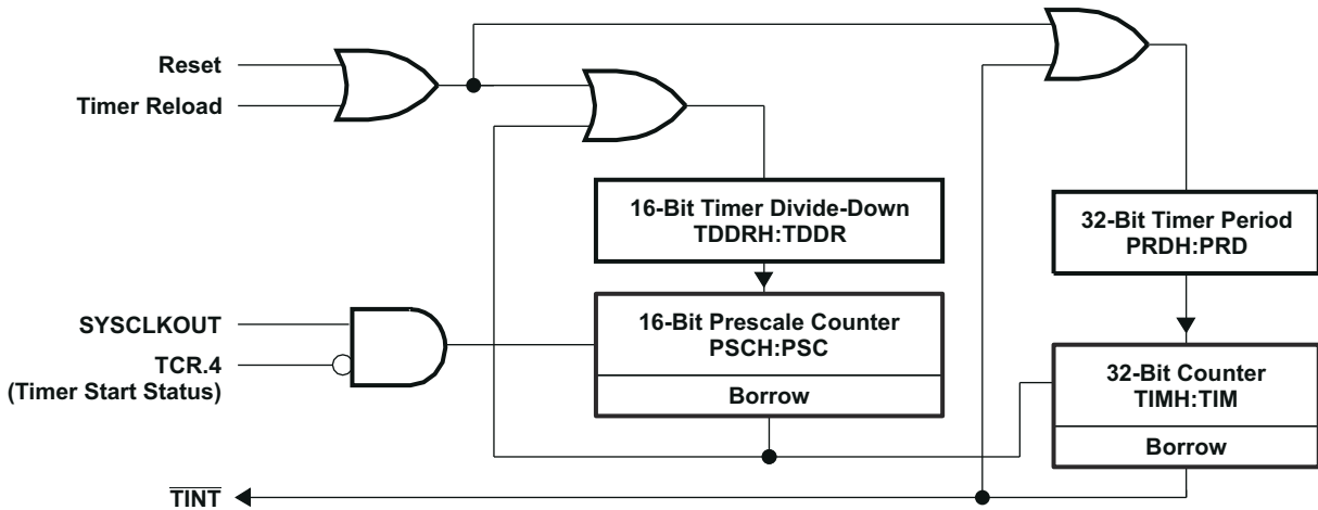
图 8-2. CPU 计时器
