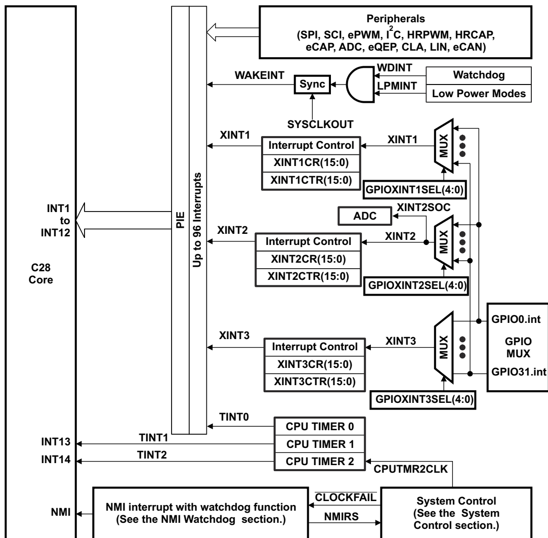
图 8-12. 外部和 PIE 中断源
