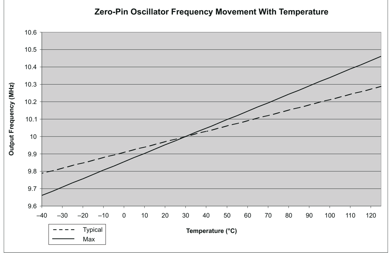
图 7-9. 随温度变化而变化的零引脚振荡器频率
