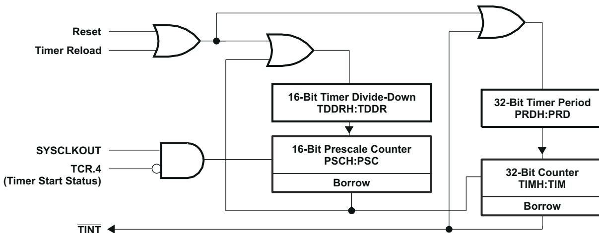
图 8-2. CPU 计时器
