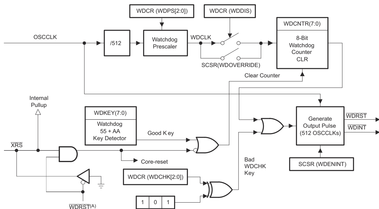
图 8-34. 看门狗模块
